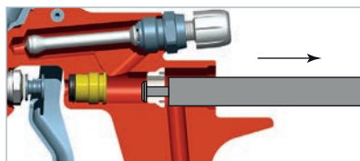
Desmontaje Fig.13.1
